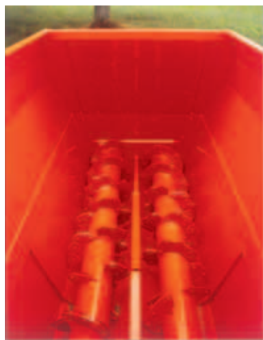
Fig.2 - Transportadores sem-fime contra-faca
